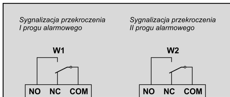
Rys.3. Schemat wyjść stykowych (przełącznikowych) detektora „uniTOX.CO K”
