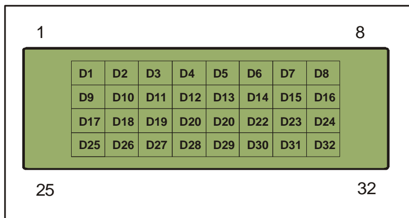
Rys.2 Wyświetlacz LCD – podział na pola informujące o stanie detektorów
