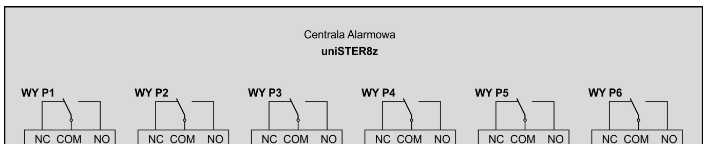
Rys.5. Schemat wyjść stykowych (przekaźnikowych) Centrali Alarmowej uniSTER8z
